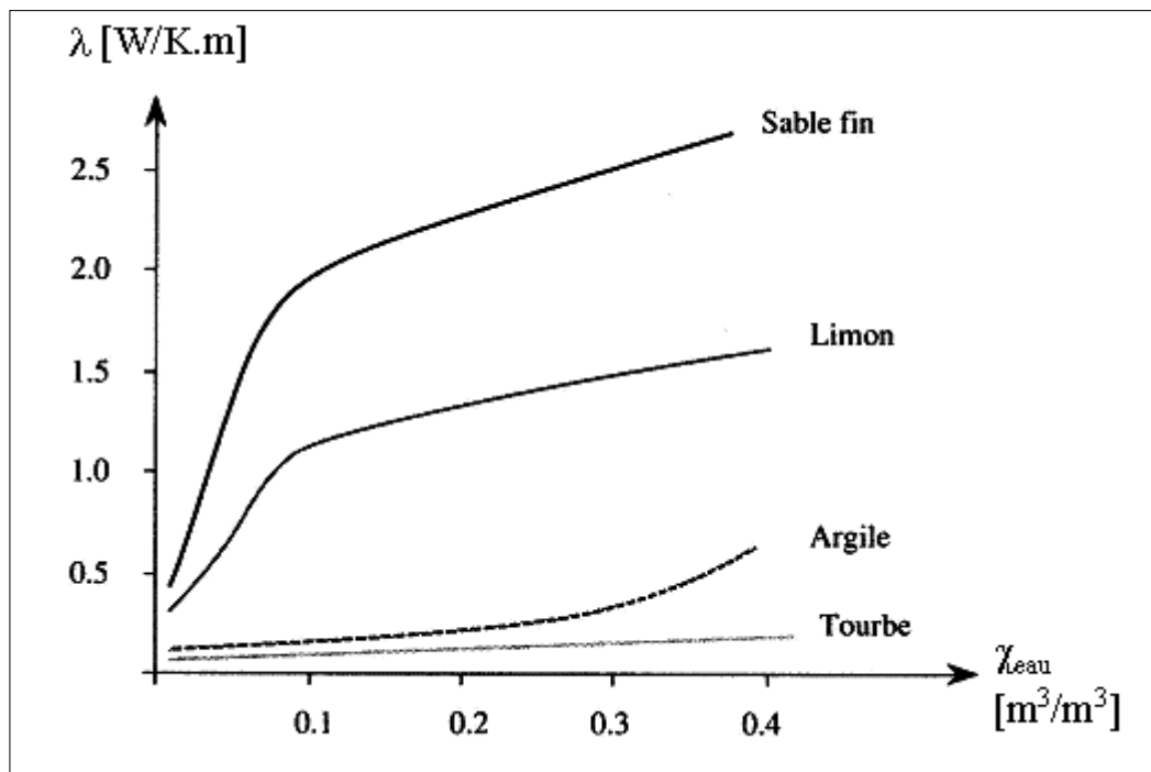
Conductivité thermique \lambda de quelques sols en fonction de la teneur en eau
